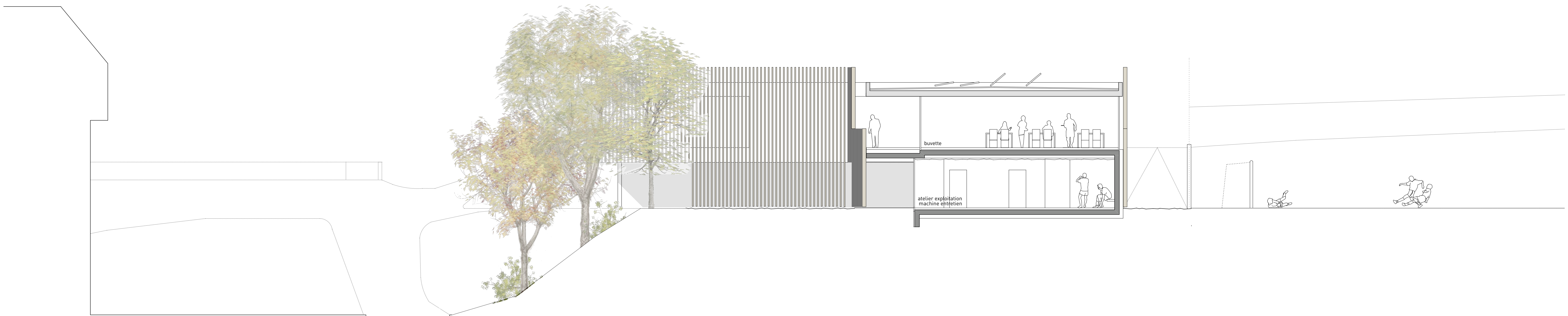
coupe Nord-Sud 1/100
